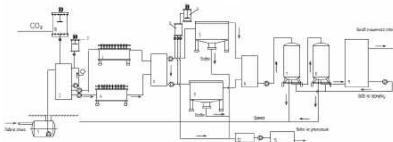
Рисунок 1 – Схема очистки сточных вод локомотивного депо
