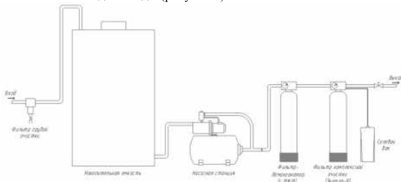
Рисунок 1 – Схема водоочистной установки
