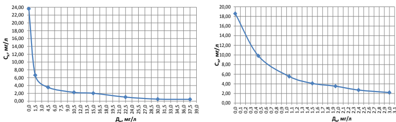
Рисунок 2 – Зависимость снижения мутности обрабатываемой промывной воды от дозы коагулянта
