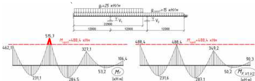
Рисунок 3 – Реализация управления при эксплуатации конструкции с постоянными и временными воздействиями: а) расчетная схема балки с регуляторами; б) эпюры изгибающих моментов; в) с регулированием
