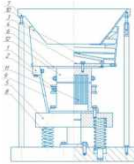
Рисунок 6 – Вибробункер
